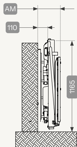
Plateforme repliée avec fixation au mur
