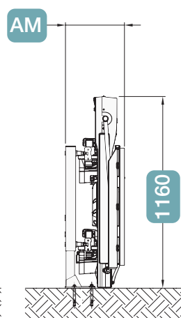
Plateforme repliée
