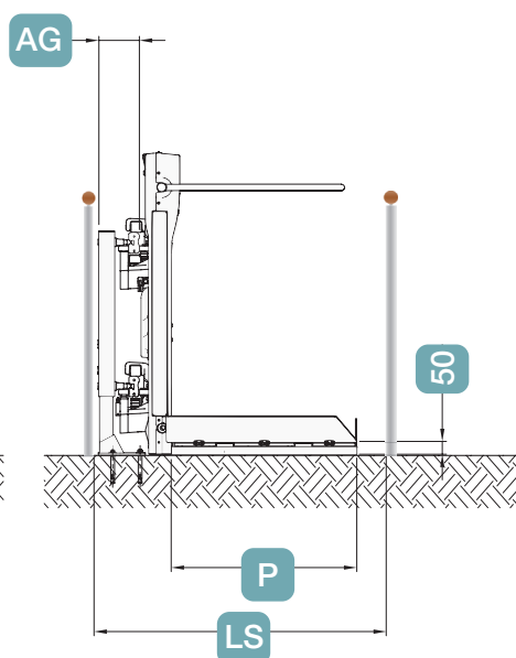
Plateforme dépliée
