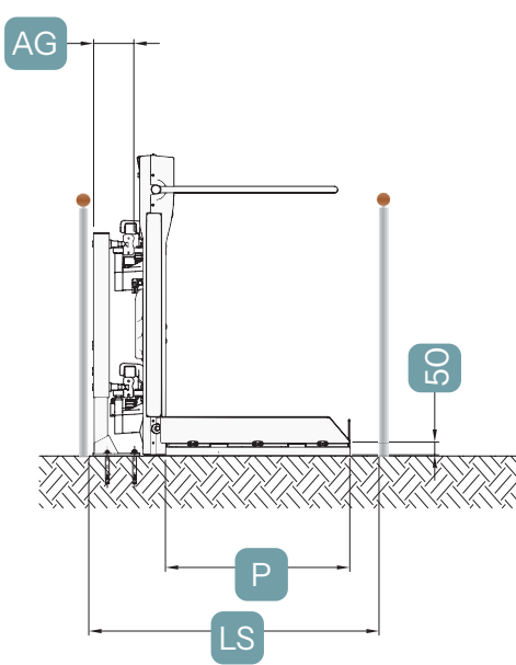
Ungeklappte Plattform
