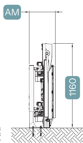
Geklappte Plattform
