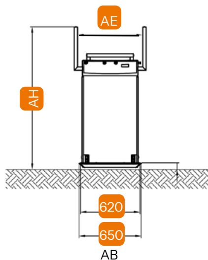
Plateforme totalement dépliée (entrée/sortie à l'étage inférieur)
