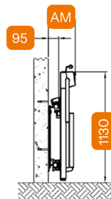
Eingeklappte Plattform mit Befestigung an die Wand
