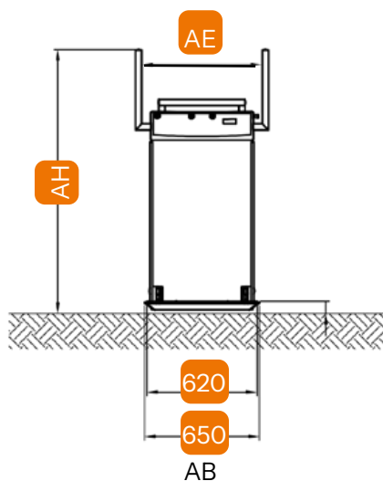
Aufgeklappte Plattform (Ein- und Aussteigen an der unteren Etage)
